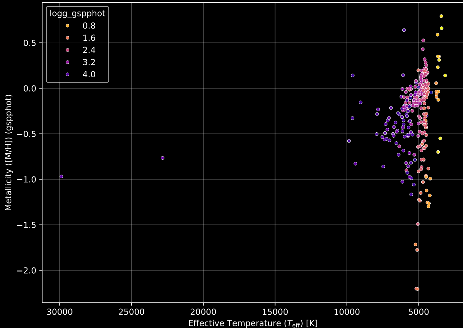
APOGEE DR17 Field: [SGRC3] Stellar Population Parameters (n= 308)
